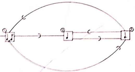
Graphe talea 1
